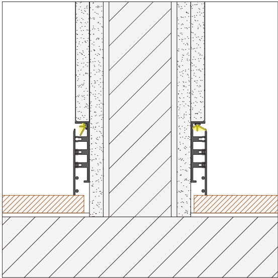
Perfis em alumínio de encaixe rápido com diferentes tipos de aplicação. Preparados para receber fita de LED de 5mm. Medida máxima fornecida 2700 mm (fita de LED não fornecida)
