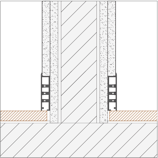
Perfis em alumínio de encaixe rápido com diferentes tipos de aplicação. Medida máxima fornecida 2700 mm *
