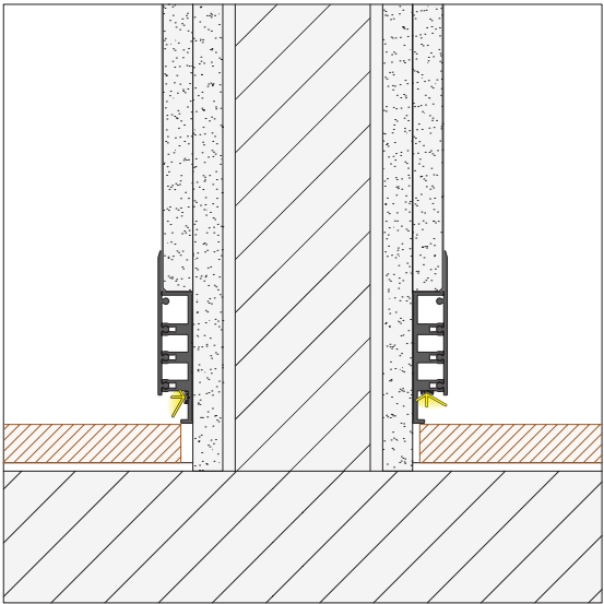
Perfis em alumínio de encaixe rápido com diferentes tipos de aplicação. Preparados para receber fitas de LED de 5mm. Medida máxima fornecida 2700 mm (fita de LED não fornecida)
